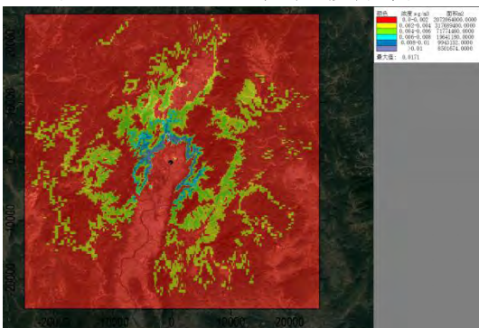
图 6.2.3.6-27 Ni 小时浓度分布图
