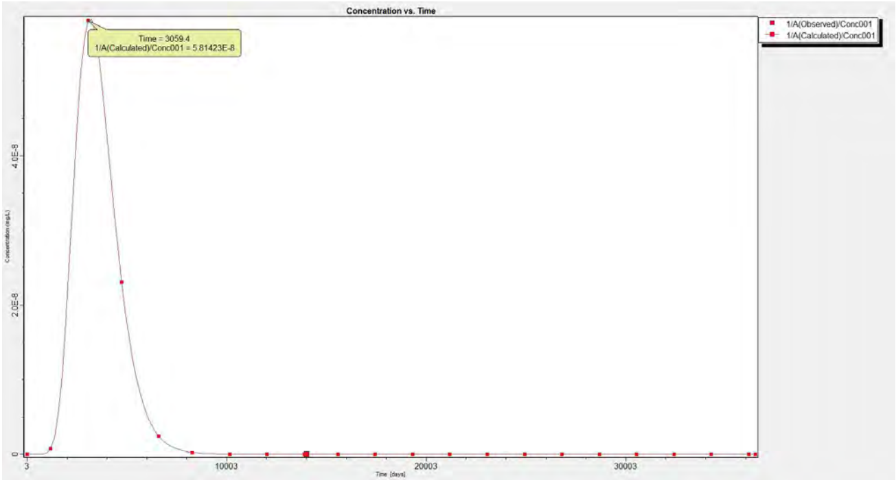
图 6.2.2.2-16 一级水洗反应器泄漏后观测井镉浓度随时间变化情况
