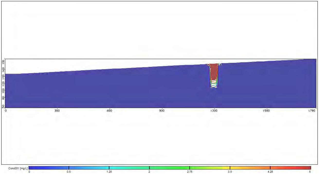
图 6.2.2.2-27 泄漏事故发生 3 天后耗氧量剖面浓度分布情况图
