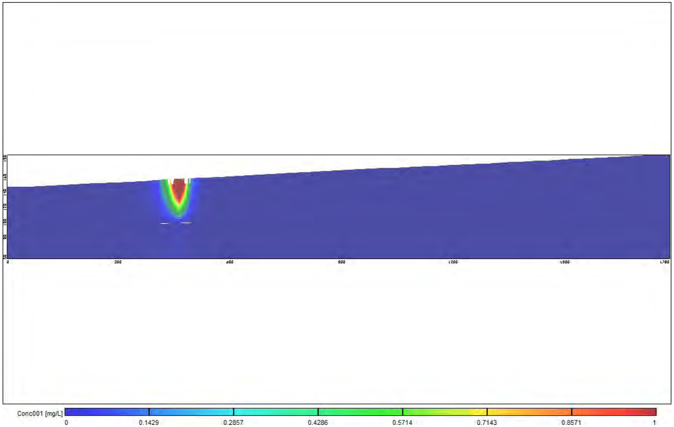
图 6.2.2.2-120 泄漏事故发生 100 天后氨氮剖面浓度分布情况图
