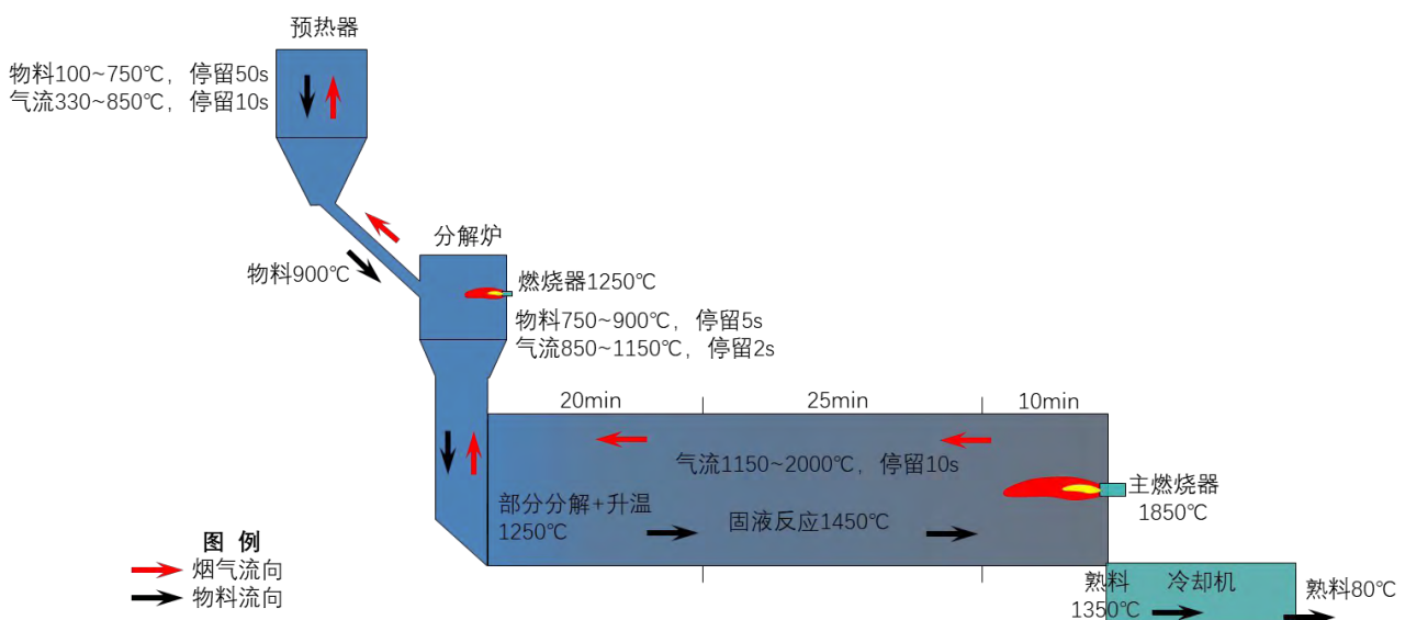
图 4.2.5.1-1 新型干法水泥旋窑煅烧过程气相、固相温度分布和停留时间
