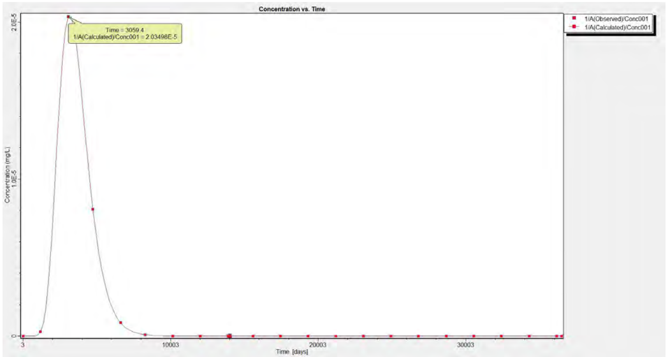
图 6.2.2.2-12 一级水洗反应器泄漏后观测井铬浓度随时间变化情况
