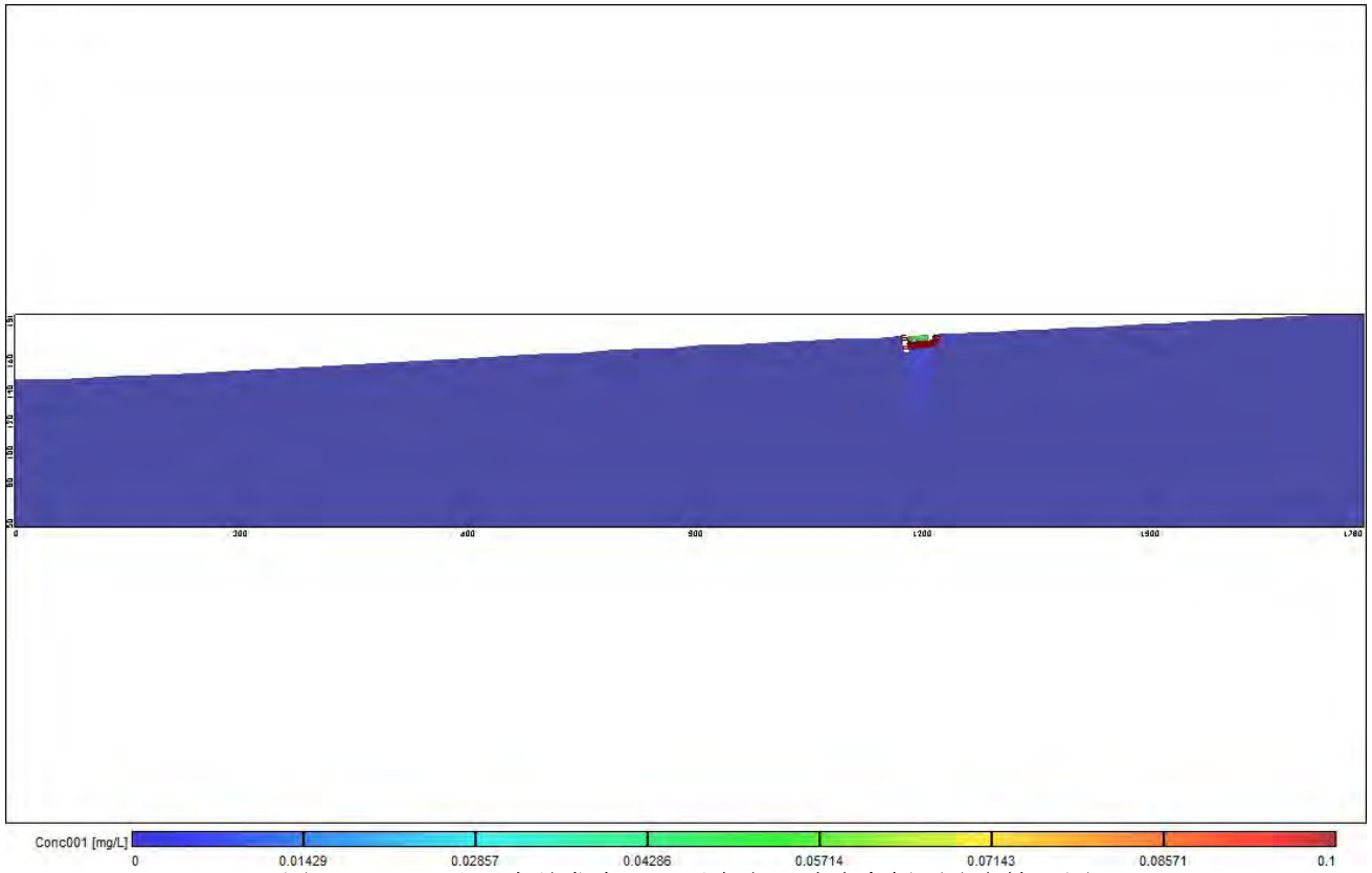
图 6.2.2.2-81 泄漏事故发生 3 天后含水层砷浓度剖面分布情况图
