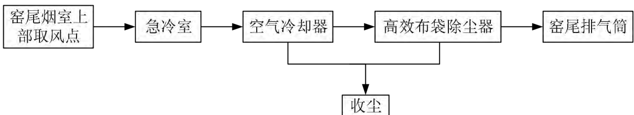
图 4.2.5.4-2 旁路放风系统的工艺流程图
