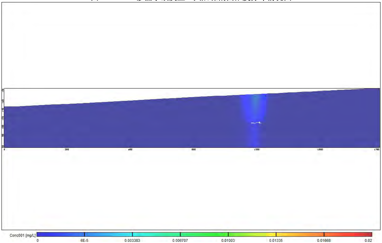
图 6.2.2.2-61 渗漏事故发生 100 天后镍剖面浓度分布情况图
