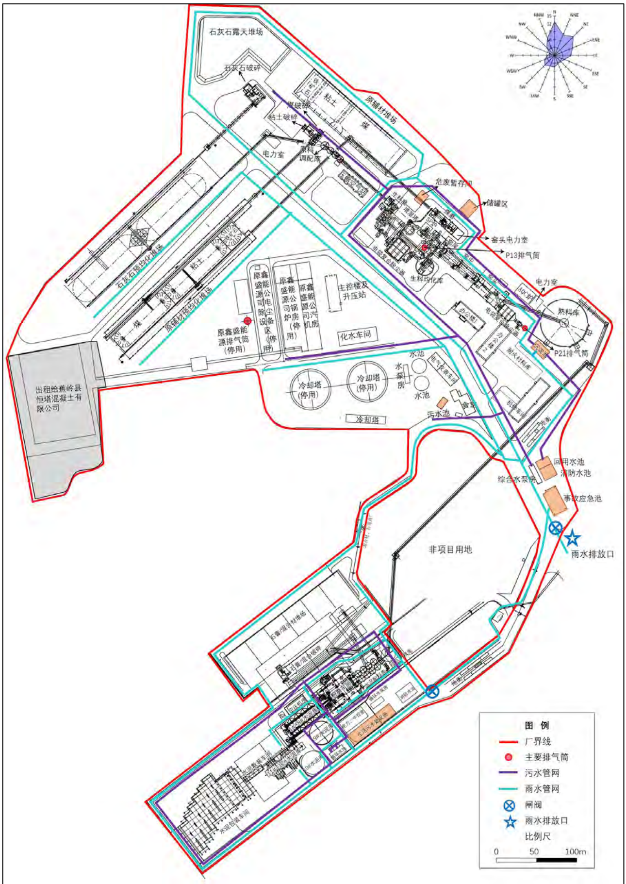
图 3.1.4-1 现有项目总平面布置图
