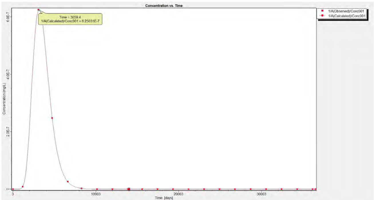
图 6.2.2.2-13 一级水洗反应器泄漏后观测井镍浓度随时间变化情况
