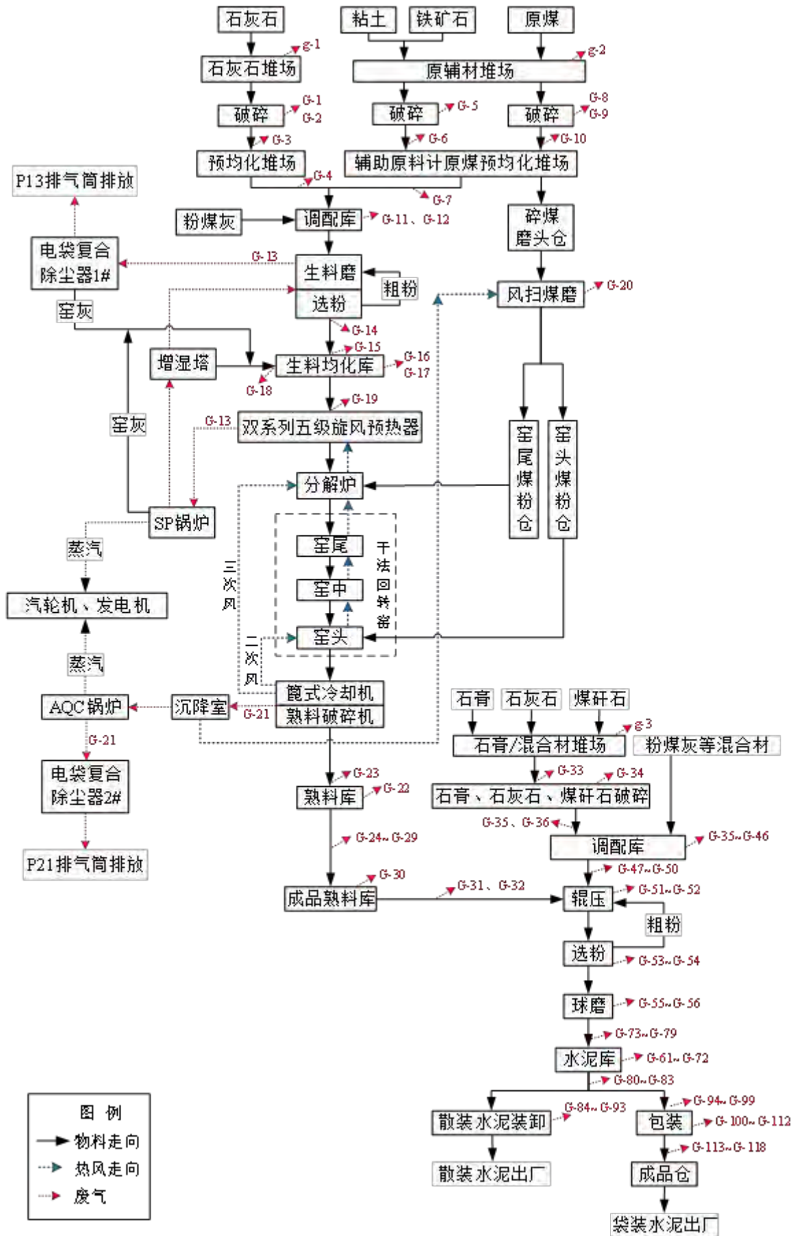
图 3.2.1-1 现有项目水泥生产工艺（熟料线+粉磨站）流程图
