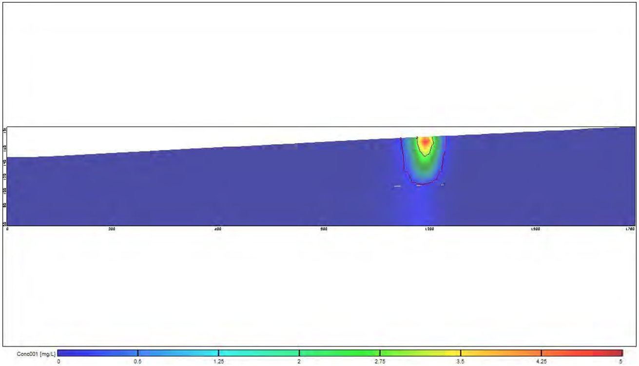
图 6.2.2.2-29 泄漏事故发生 365 天后耗氧量剖面浓度分布情况图
