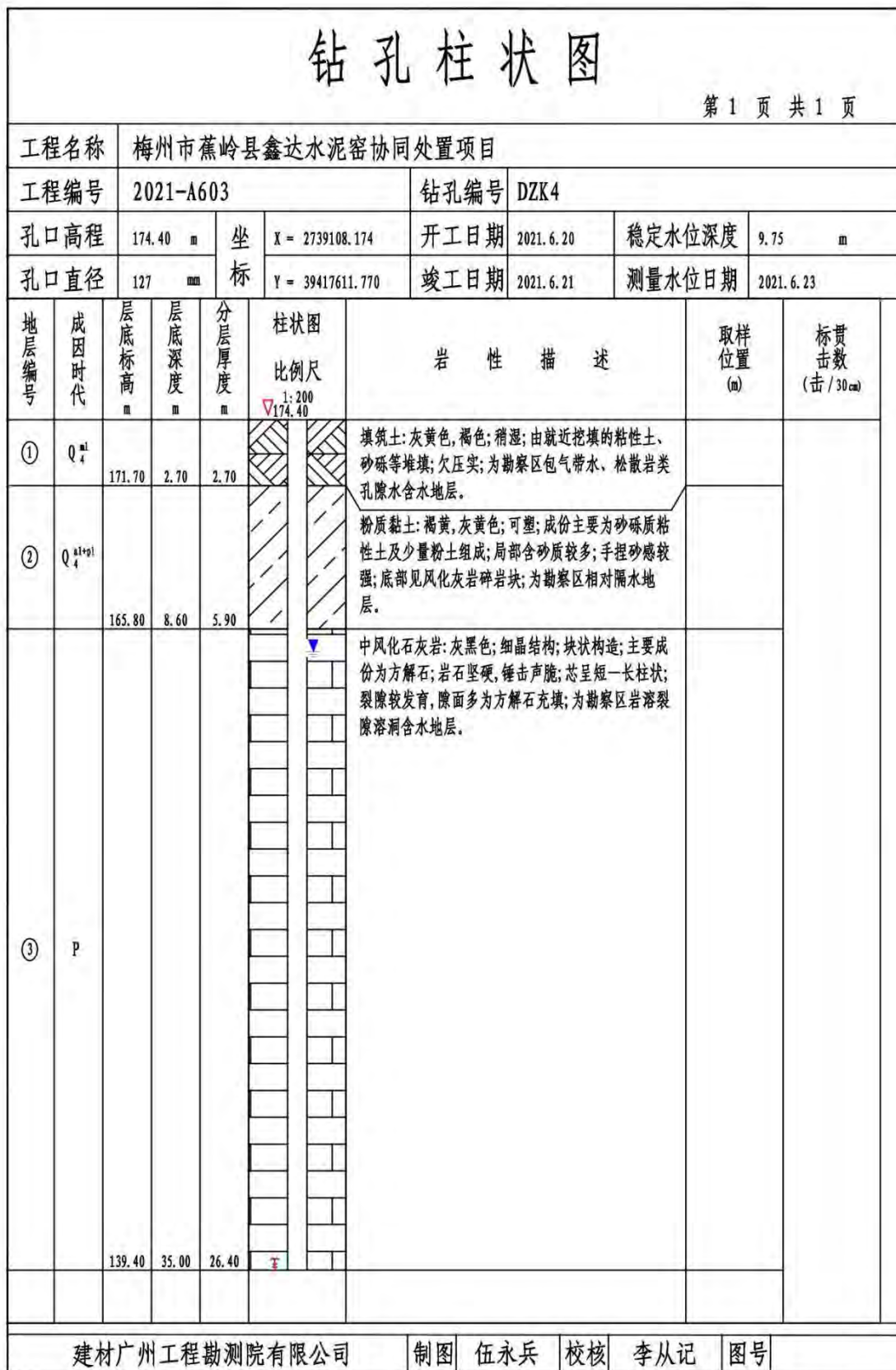
图 6.2.2.1-12 本项目钻孔柱状图
