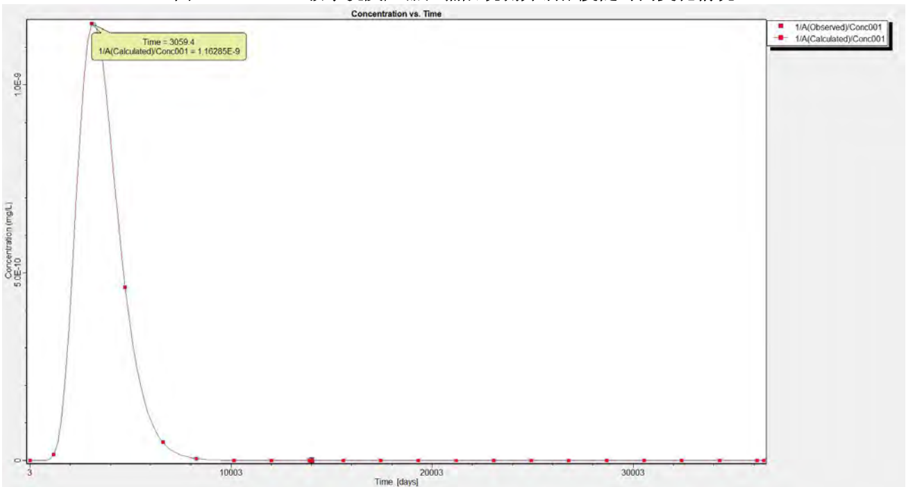
图 6.2.2.2-17 飞灰预处理车间的一级水洗反应器泄漏后观测井汞浓度随时间变化情况
