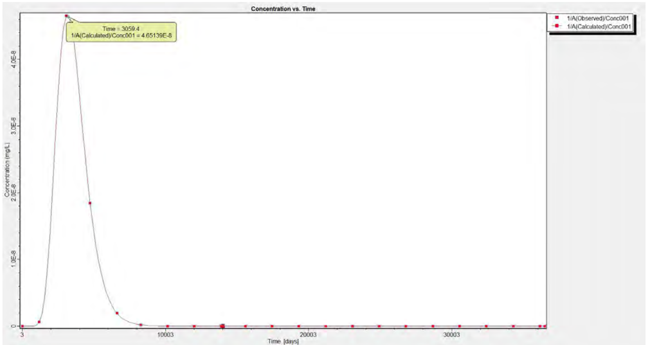
图 6.2.2.2-18 飞灰预处理车间的一级水洗反应器泄漏后观测井锰浓度随时间变化情况 B 生活污水处理设施发生泄漏事故
