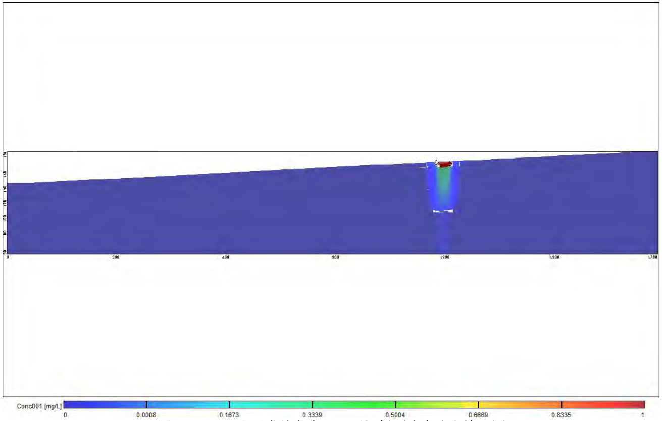
图 6.2.2.2-70 泄漏事故发生 3 天后铜剖面浓度分布情况图
