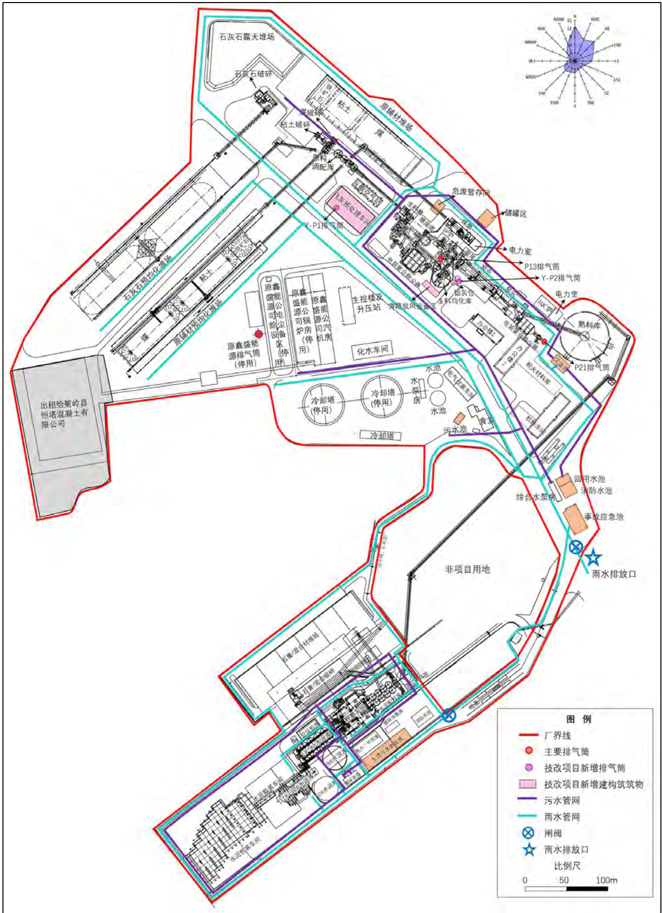
图 4.1.5-1 技改后全厂总平面布置图
