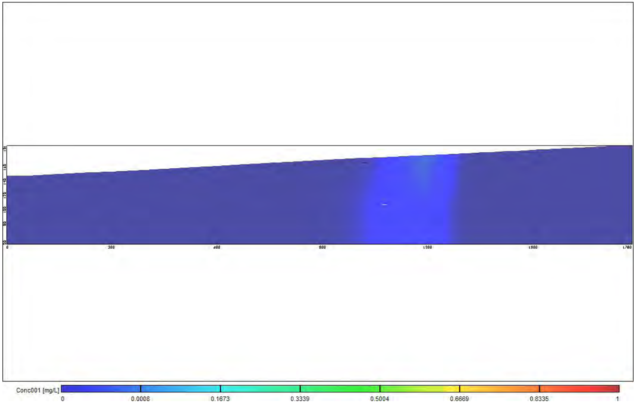
图 6.2.2.2-72 泄漏事故发生 365 天后铜剖面浓度分布情况图
