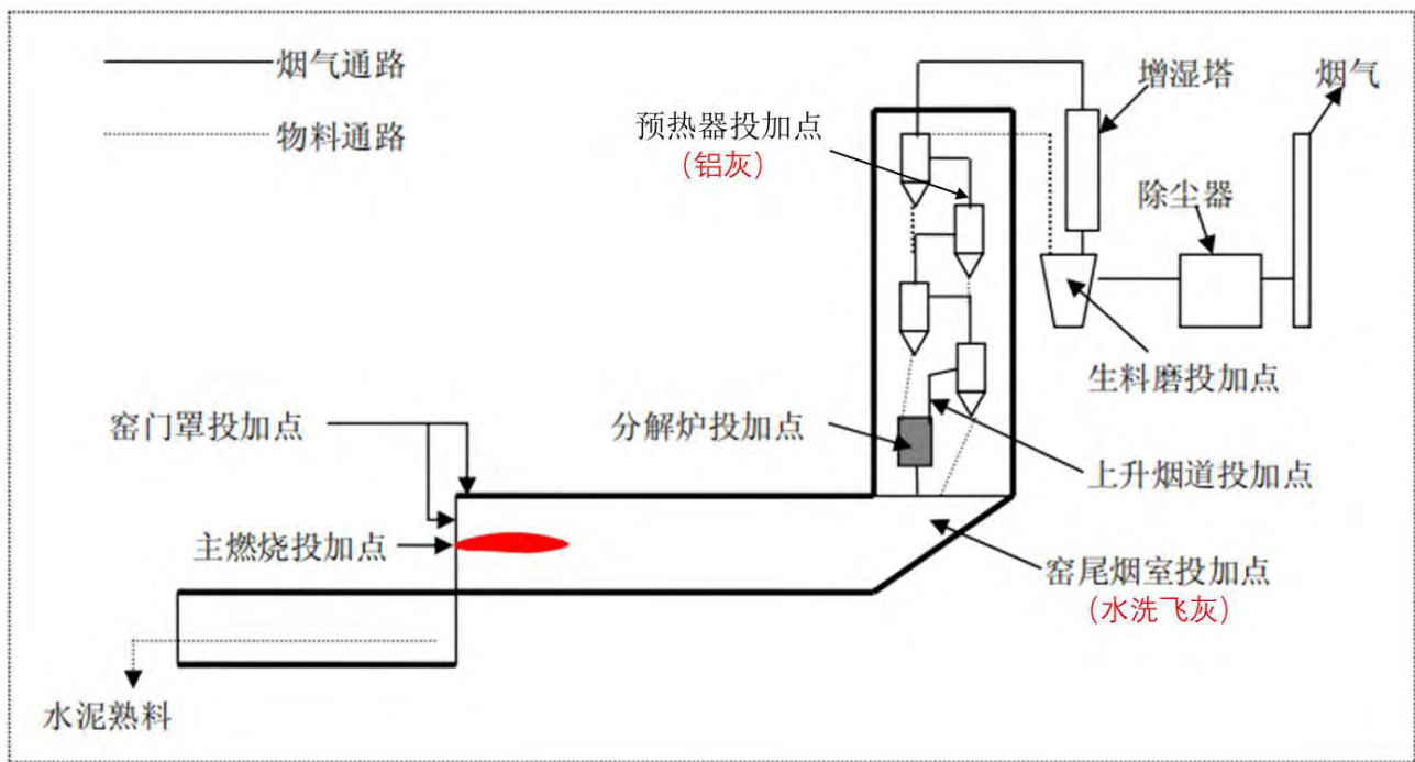
图 4.2.5.2-1 本技改项目危险废物投加口示意图
