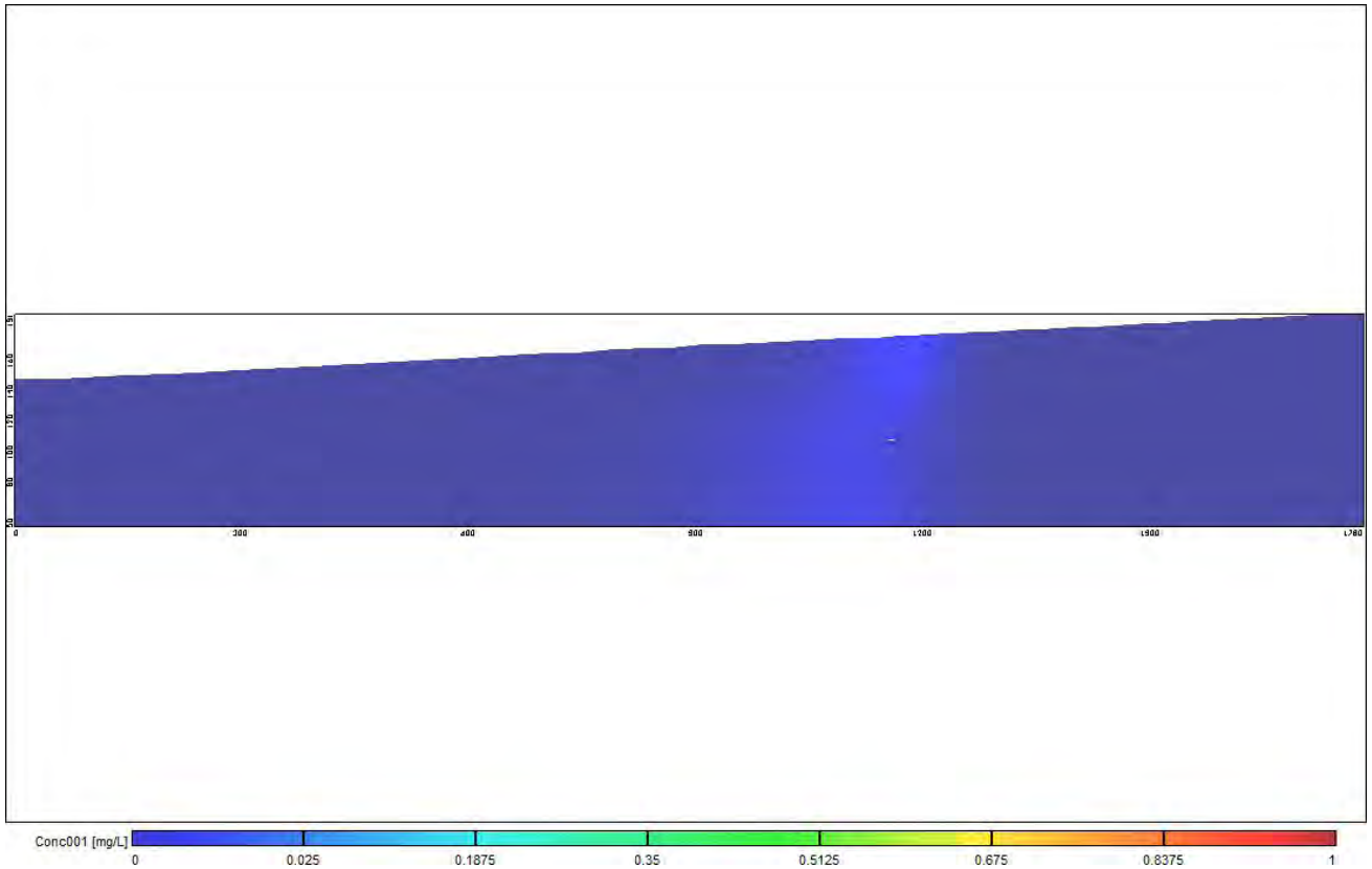
图 6.2.2.2-42 泄漏事故发生 1000 天后 NH 3 -N 浓度剖面分布情况图
