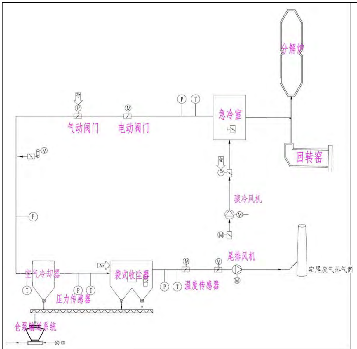
图 4.2.5.4-3 旁路放风系统的设备连接图
