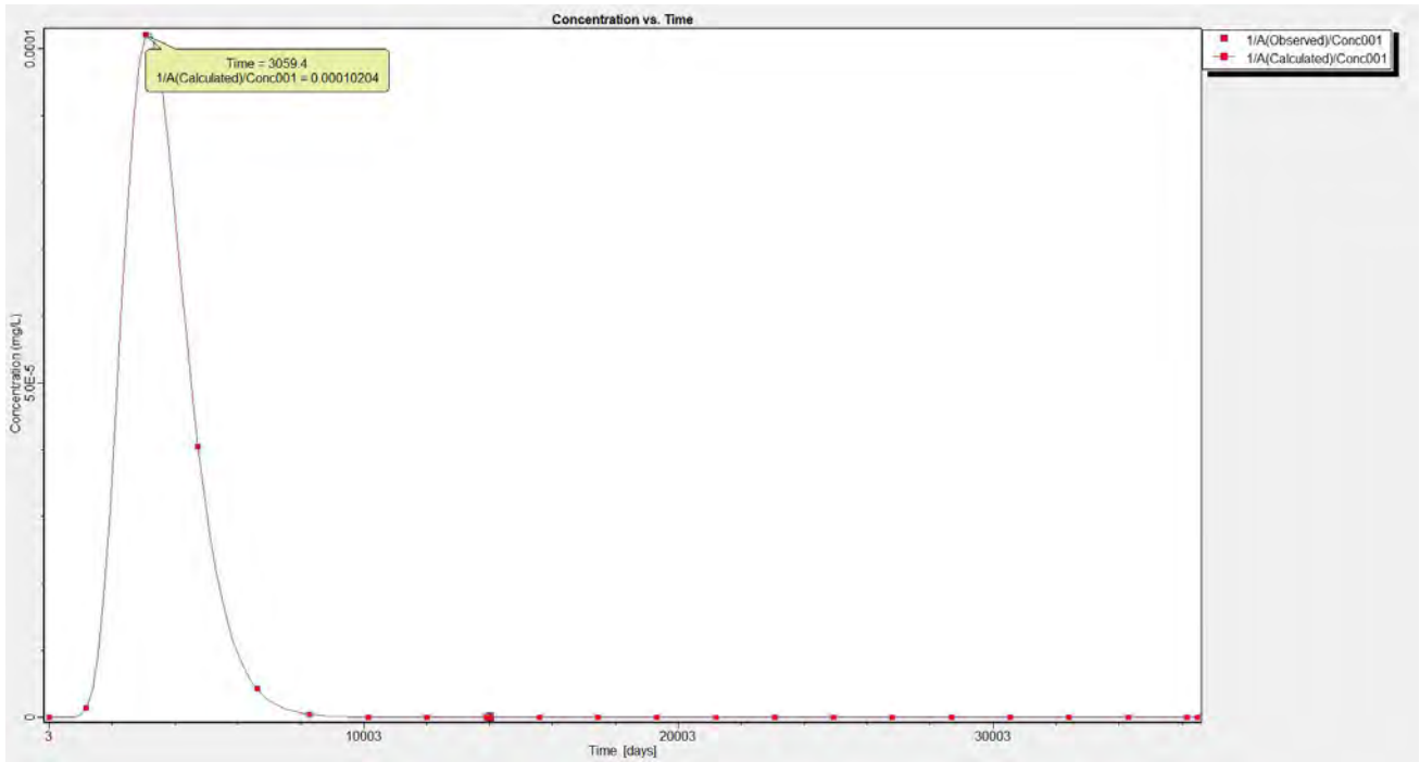
图 6.2.2.2-14 一级水洗反应器泄漏后观测井铜浓度随时间变化情况
