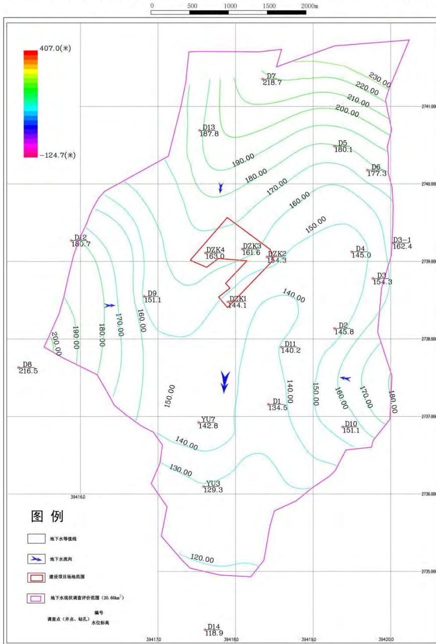
梅州市蕉岭县鑫达水泥窑协同处置项目调查评价区（枯水期）地下水等值线图
