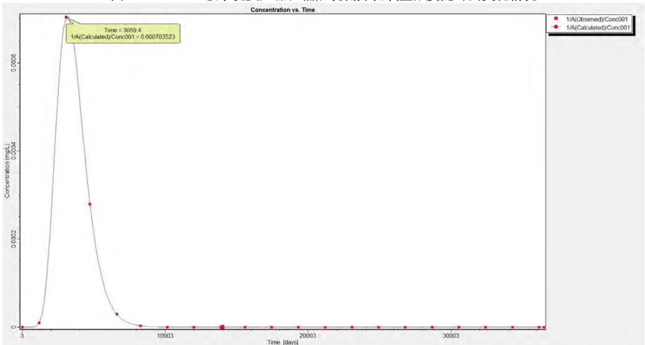
图 6.2.2.2-11 一级水洗反应器泄漏后观测井 NH 3 -N 浓度随时间变化情况
