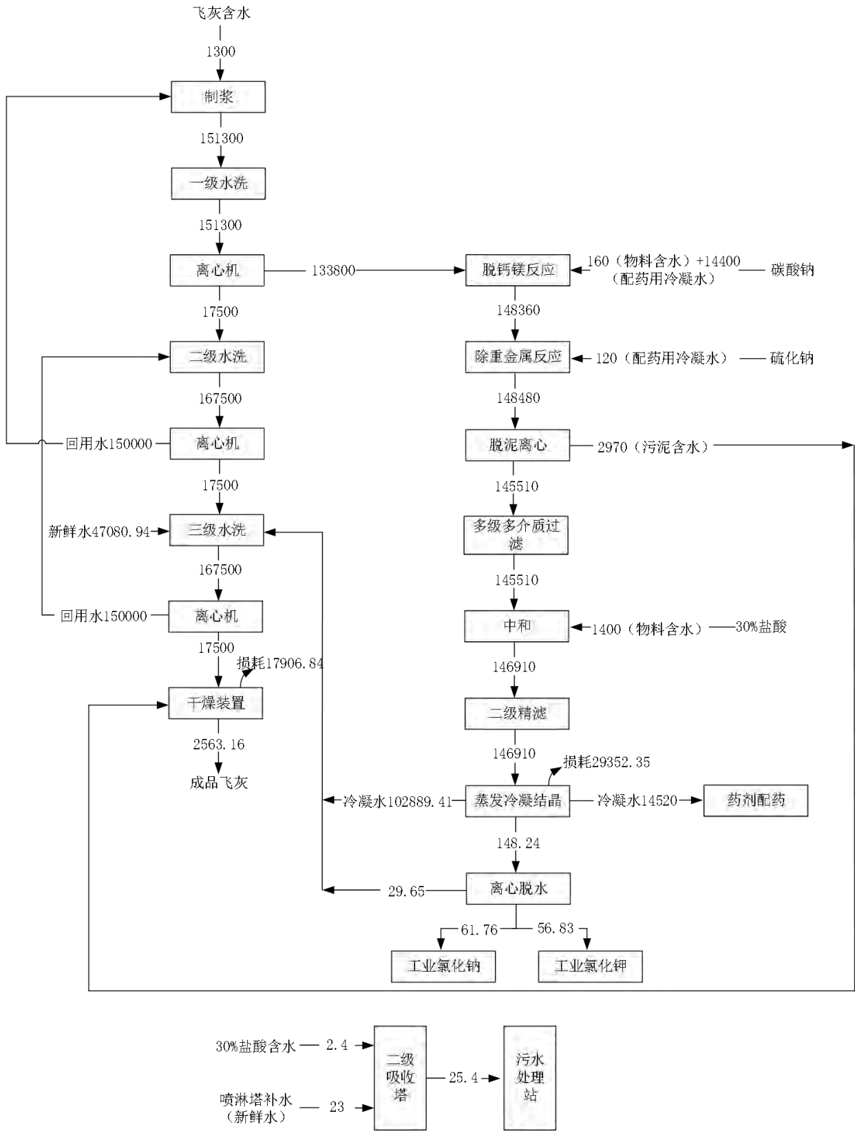
图 4.2.4.4-3 飞灰预处理车间水平衡图
